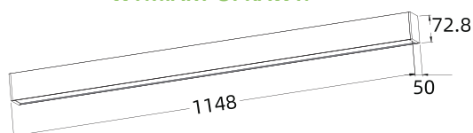
Montaż natynkowy
